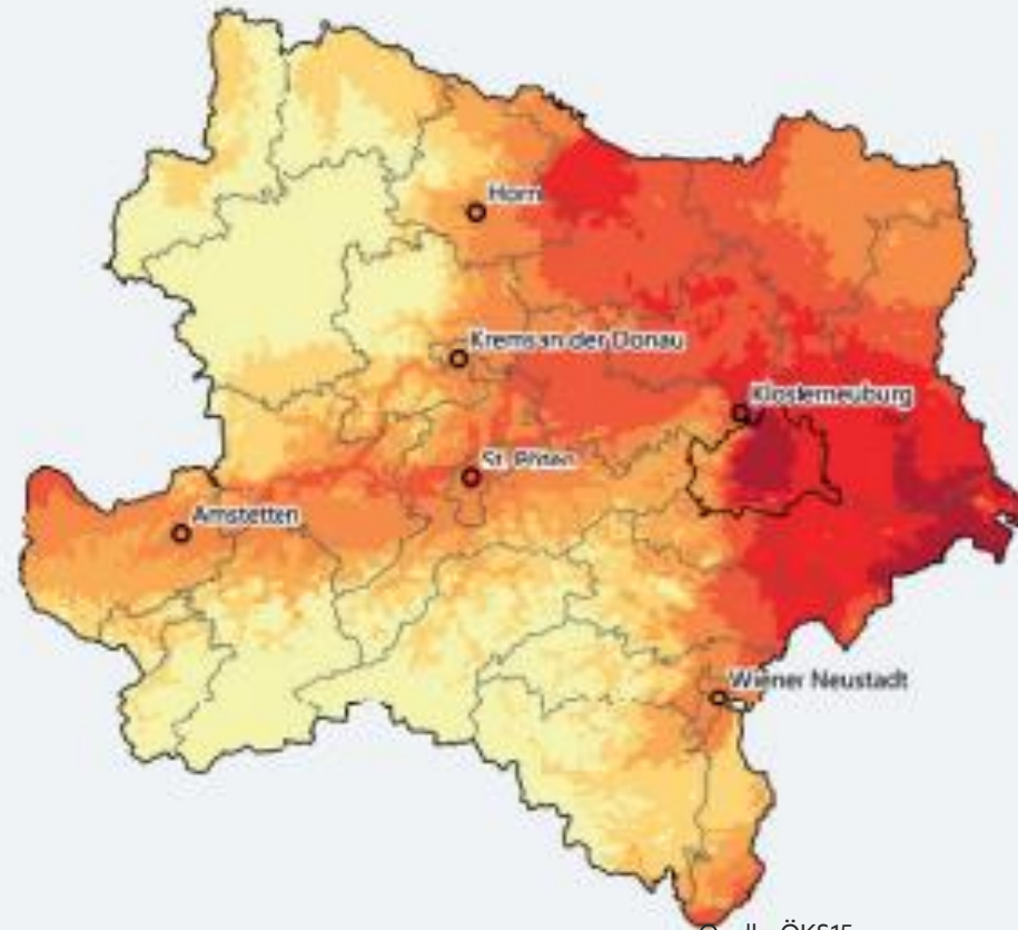
Zukünftiges Klima 2071–2100 geringe Anstrengung im Klimaschutz (RCP8.5)
